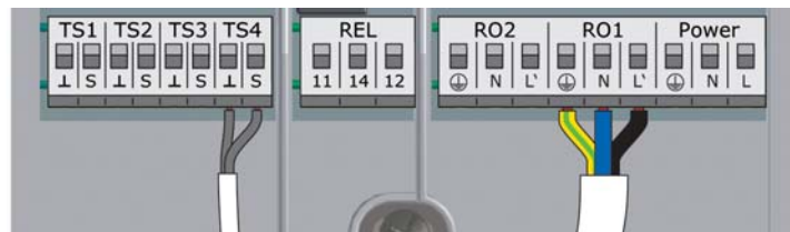
TS4: signal PWM du circulateur haut rendement Borne gauche: terre Borne droite: Signal
