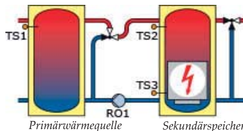
Hydraulisches Schema 2.2
