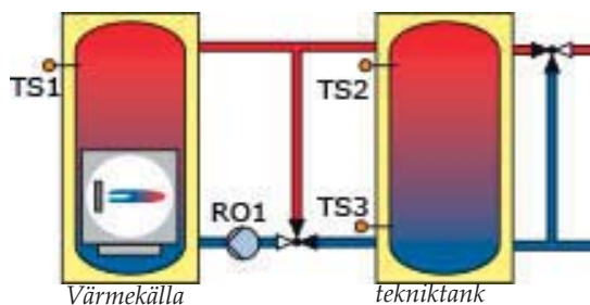
Hydraulschema 3.2
