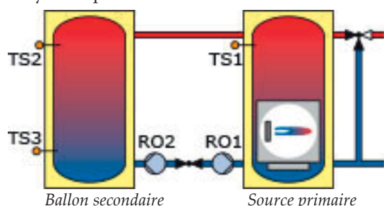
Schéma hydraulique 1.2
