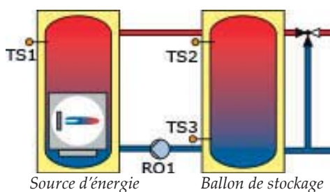
Schéma hydraulique 3.2
