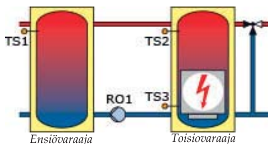
Hydraulikaavio 2.2
