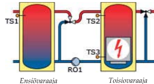
Hydraulikaavio 2.2
