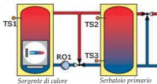
Schema idraulico 3.2
