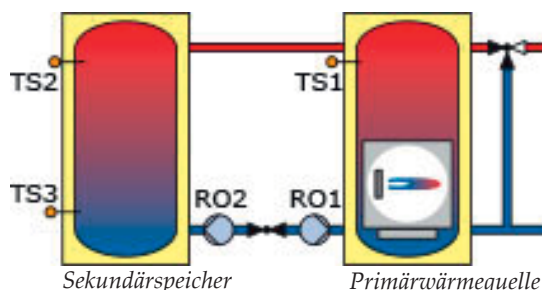
Hydraulisches Schema 1.1
