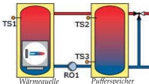
Hydraulisches Schema 3.2
