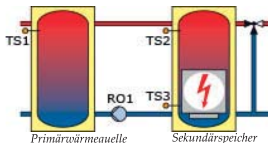
Hydraulisches Schema 2.2
