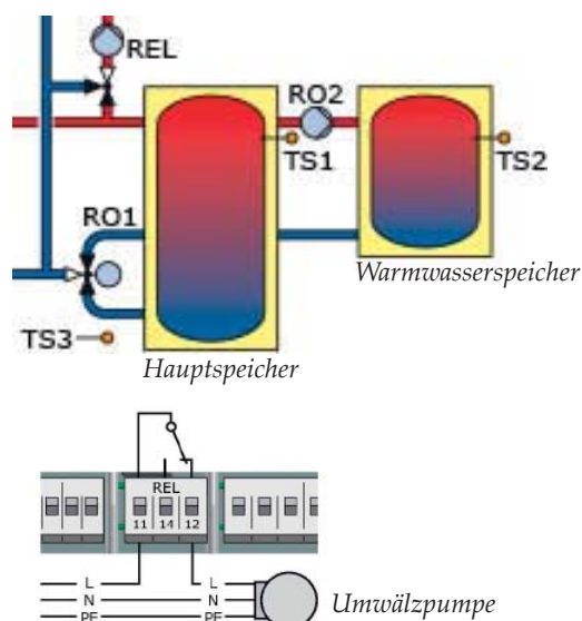
Hydraulisches Schema 4
