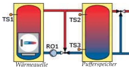
Hydraulisches Schema 3.2
