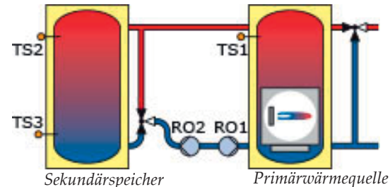
Hydraulisches Schema 1.2
