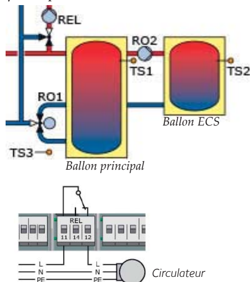
Schéma hydraulique 4
