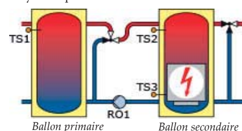
Schéma hydraulique 2.2
