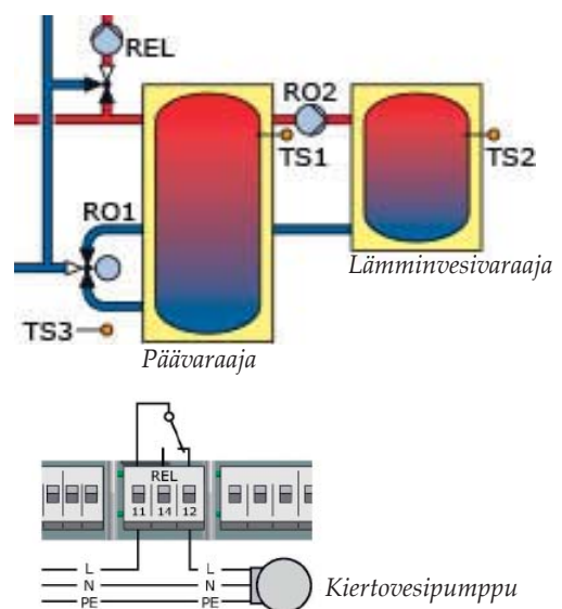
Hydraulikaavio 4
