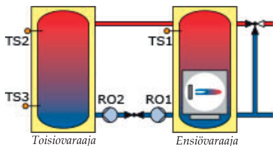
Hydraulikaavio 1.2
