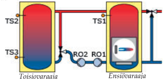
Hydraulikaavio 1.2
