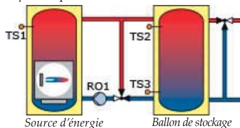
Schéma hydraulique 3.2
