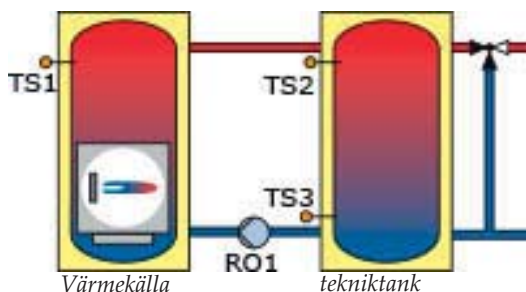
Hydraulschema 3.2
