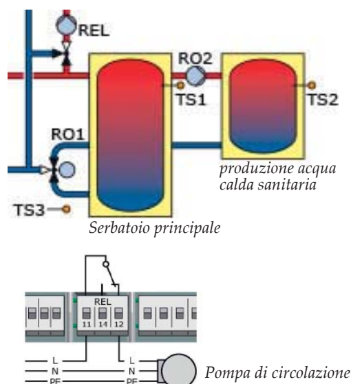
Schema idraulico 4
