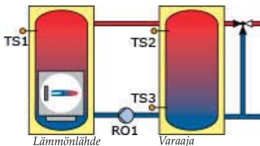
Hydraulikaavio 3.2
